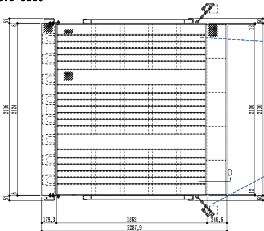
平面図
