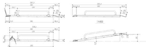
側面図
