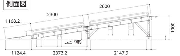
側面図
