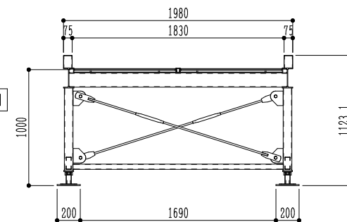
スロープ A矢视图
