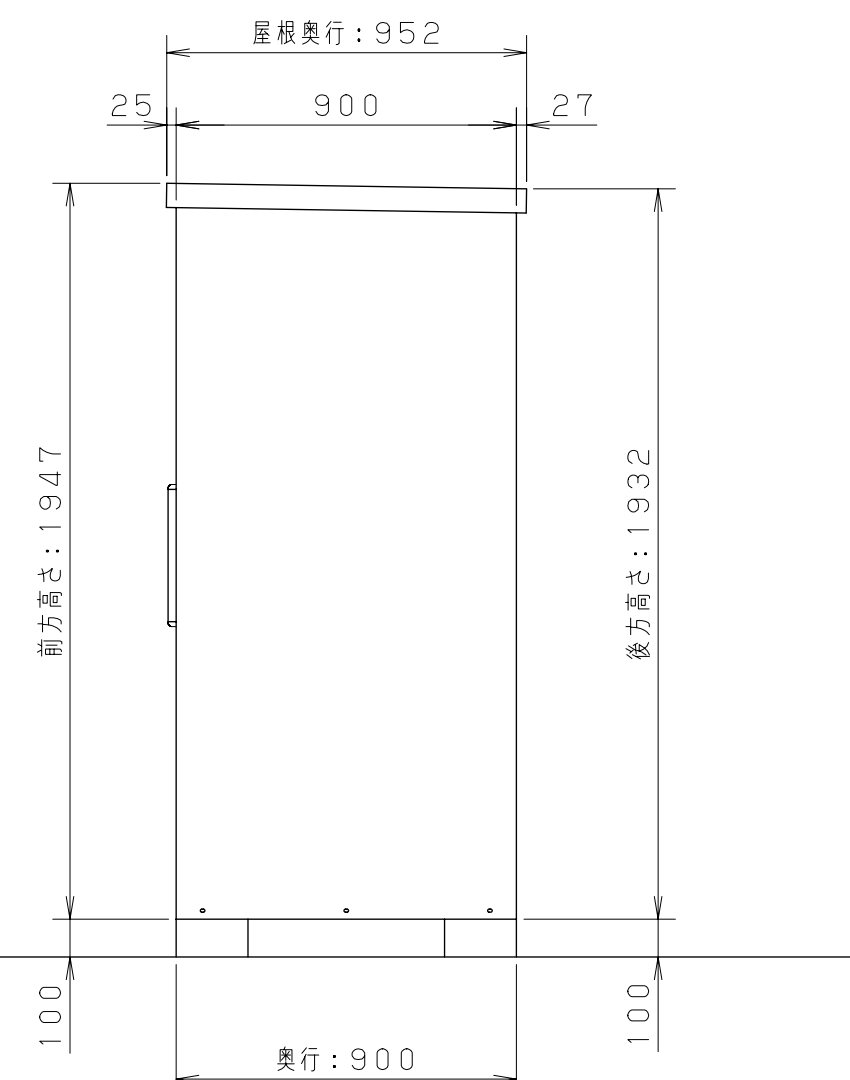
<側面図 S=1/20>
