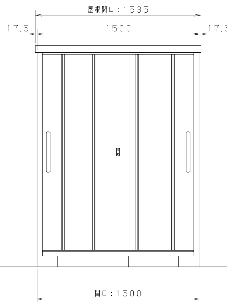
<正面図 S=1/20>
