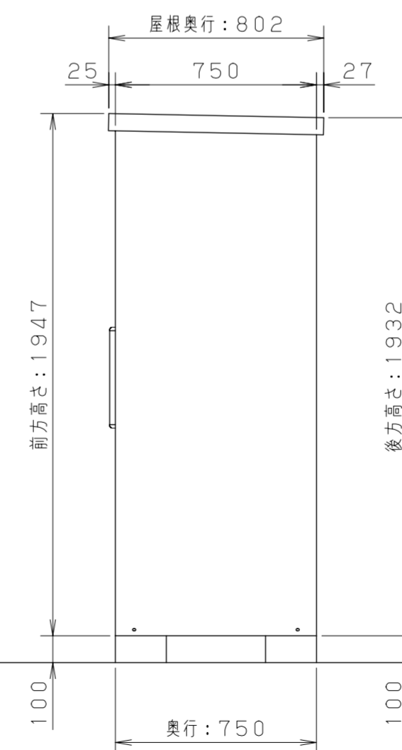
<側面図 S=1/20>
