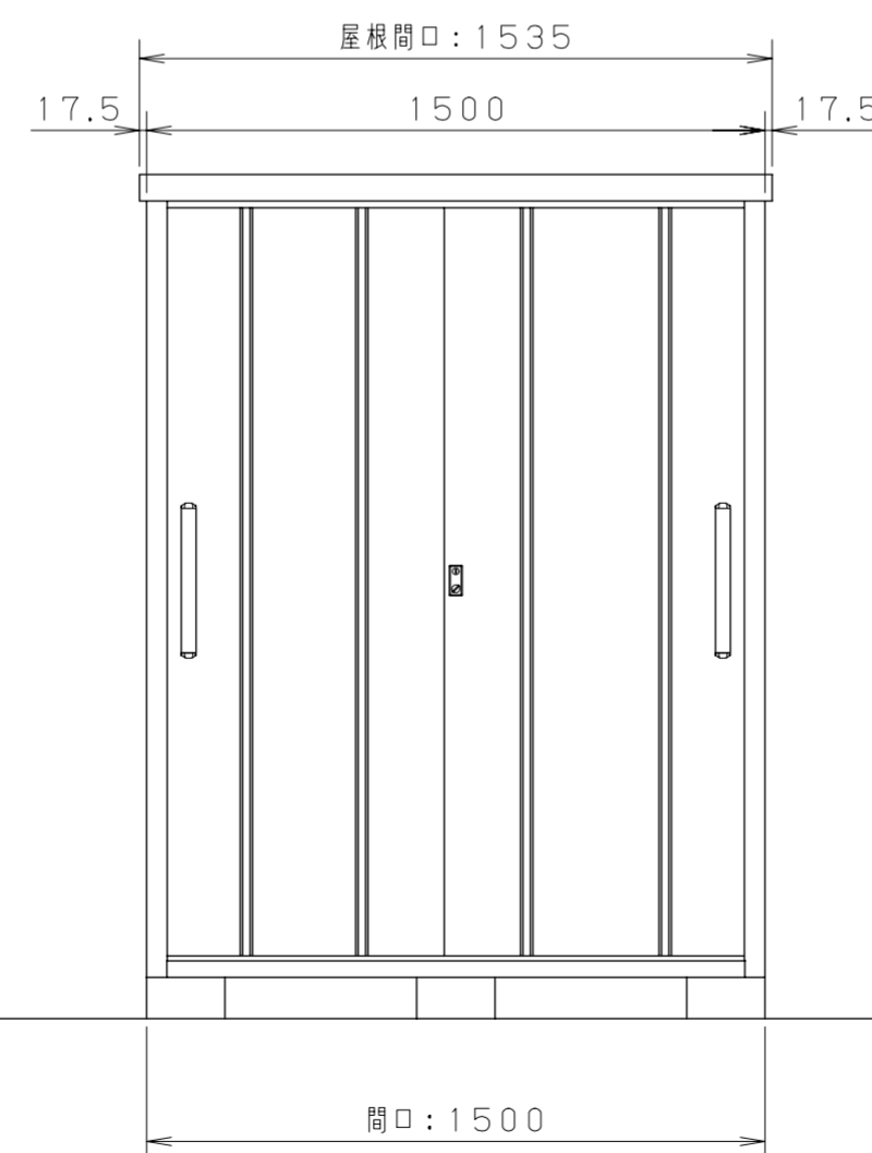
<正面図 S=1/20>
