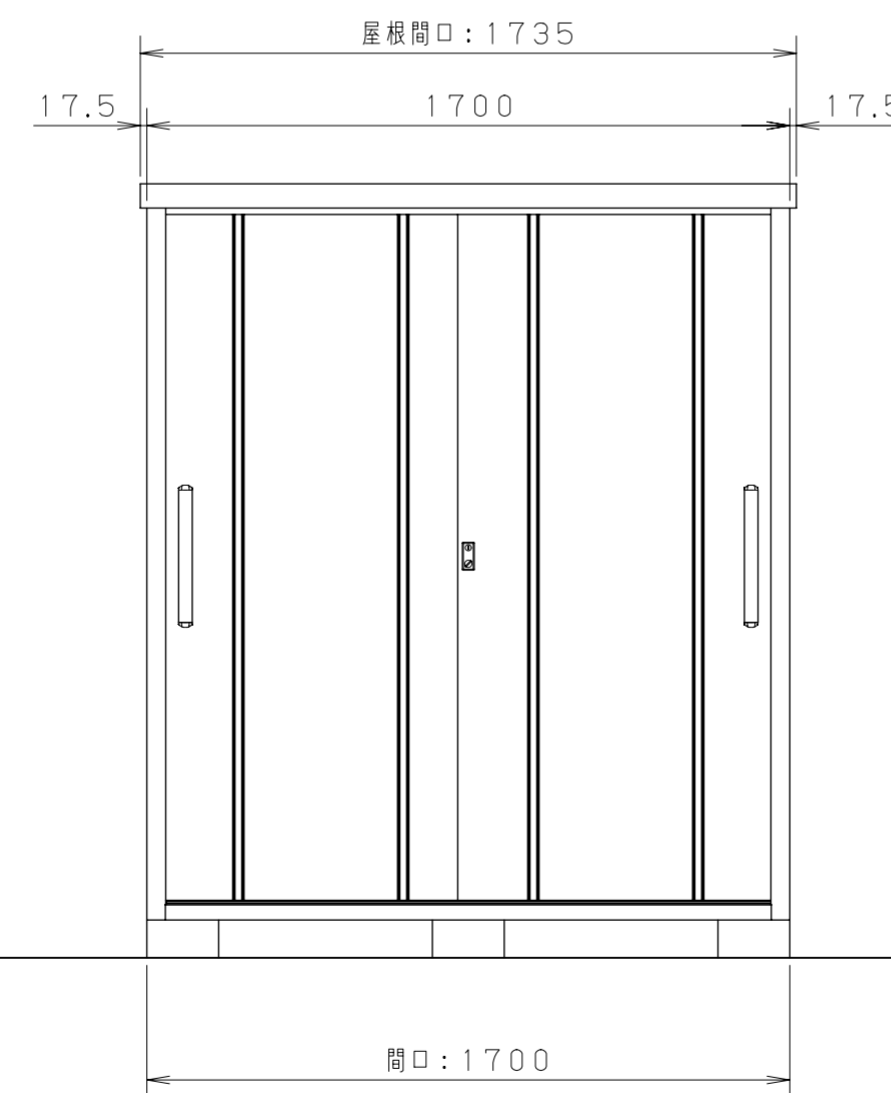
<正面図 S=1/20>
