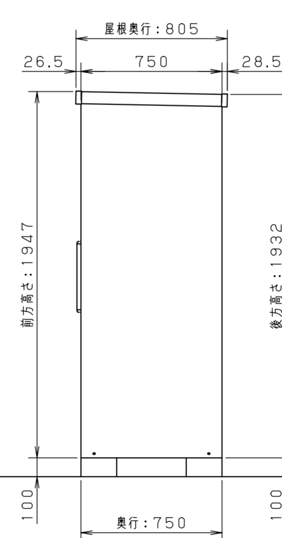
<側面図 S=1/20>
