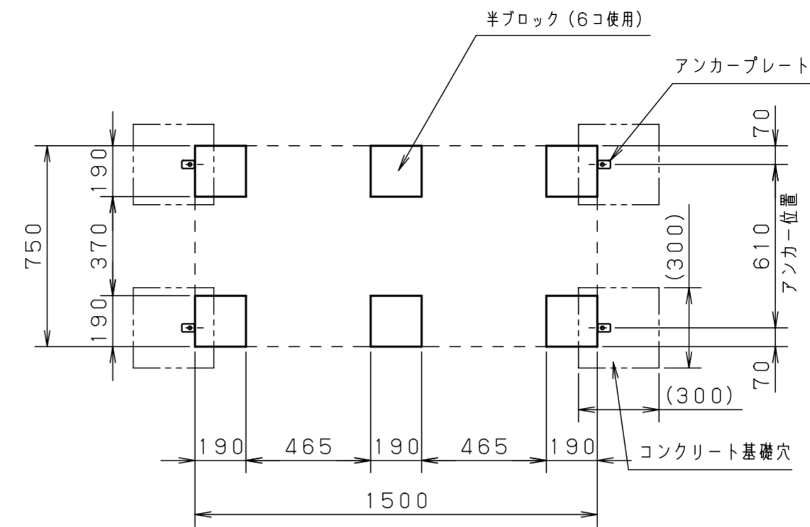
<半ブロック配置参考図>
