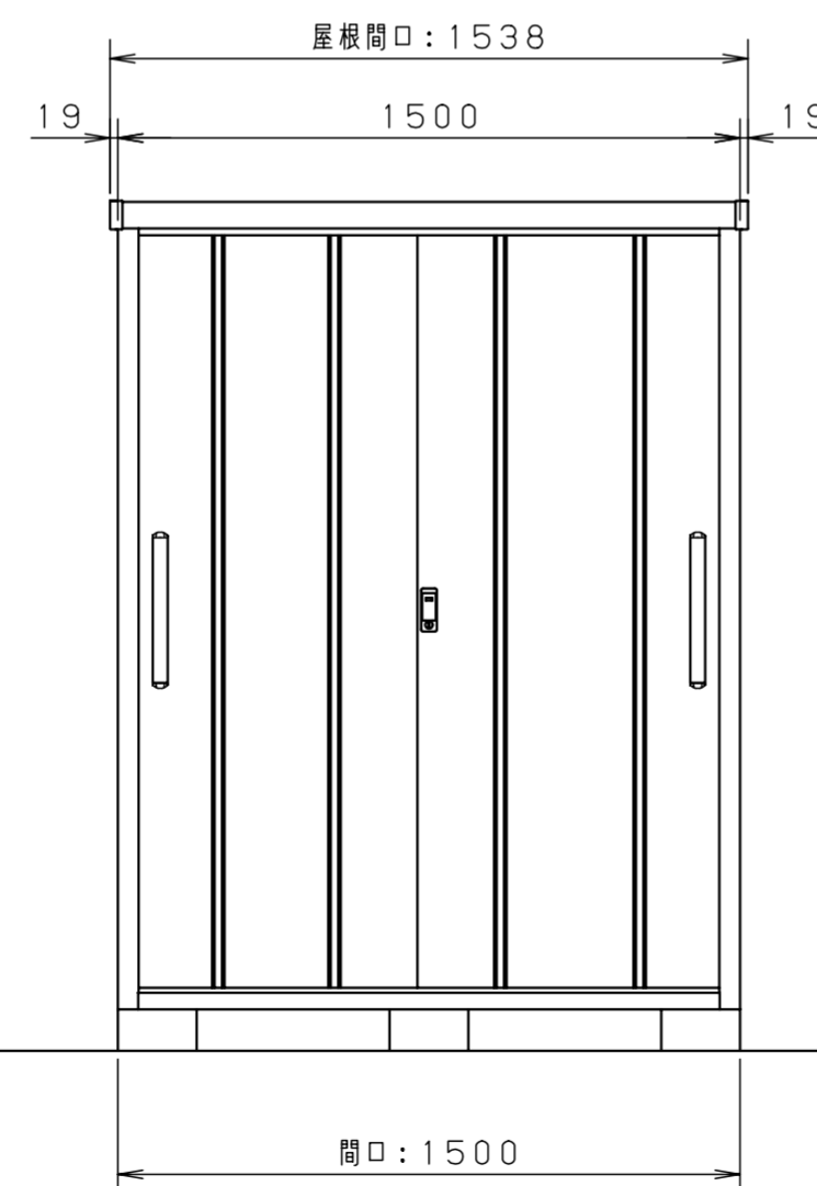
<正面図 S=1/20>
