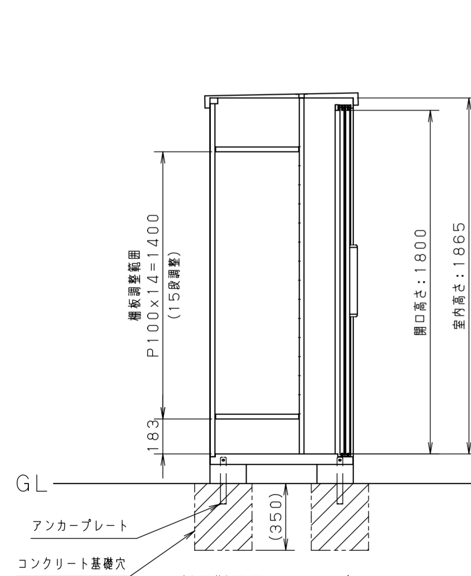
<側面断面図 S=1/20>
