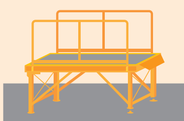
高い手すり (H:500mm H:1000mm) ※標準は200mm
