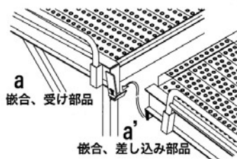
接続部
