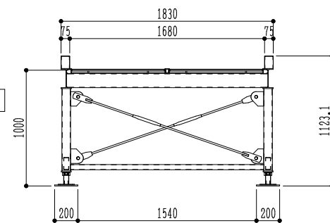
スロープ A矢視図
