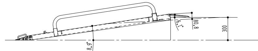
D矢視図
