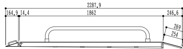
D矢視図
